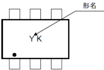
図 8.1 現品表示 RN2910FE
