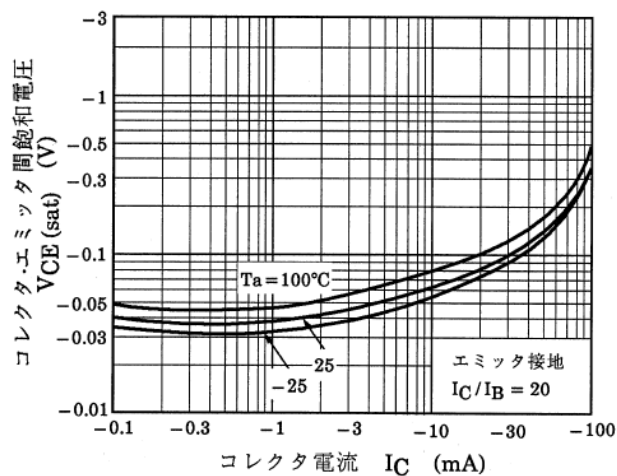
図 9.7 RN2910FE V_{CE(sat)}-I_C
