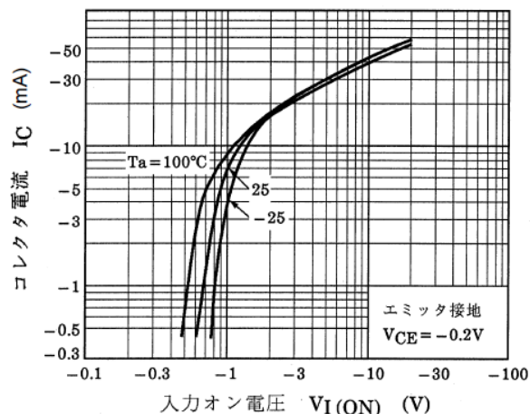
図 9.2 RN2911FE I_C - V_{I(ON)}
