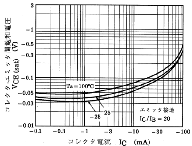
図 9.8 RN2911FE V_{CE(sat)}-I_C
