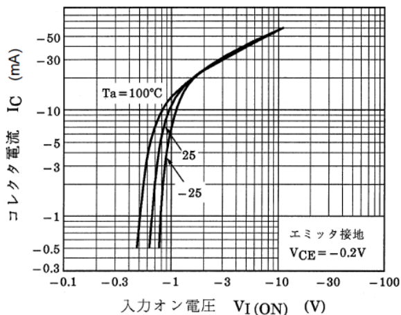
図 9.1 RN2910FE I_C - V_{I(ON)}
