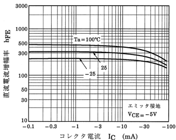
図 9.5 RN2910FE h_{FE} - I_C
