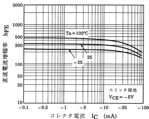
図 9.6 RN2911FE h_{FE} - I_C
