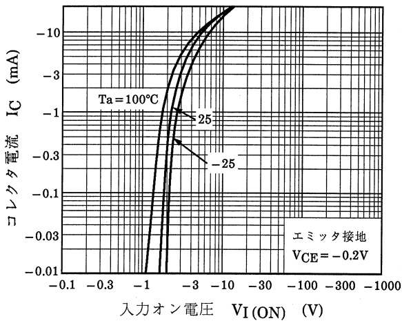
図 7.5 RN2709JE I_C - V_{I(ON)}
