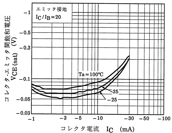
図 7.11 RN2709JE V_{CE(sat)} - I_C
