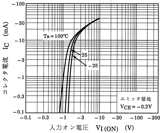
図 7.1 RN2707JE I_C - V_{I(ON)}
