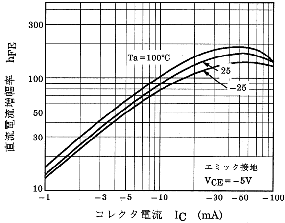
図 7.7 RN2707JE h_{FE} - I_C
