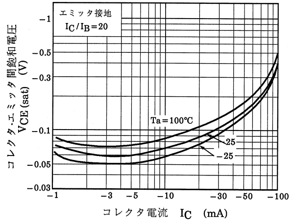
図 7.8 RN2707JE V_{CE(sat)} - I_C
