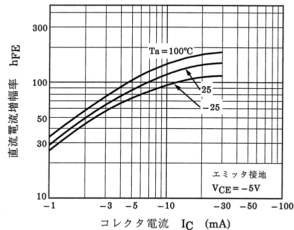
図 7.11 RN2709JE h_{FE} - I_C
