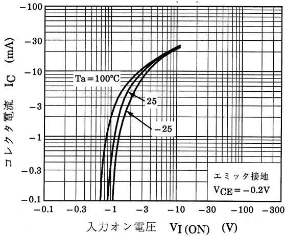
図 7.3 RN2708JE I_C - V_{I(ON)}
