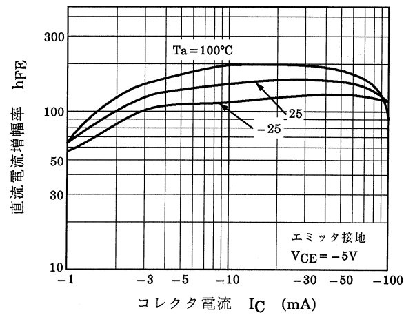
図 7.9 RN2708JE h_{FE} - I_C
