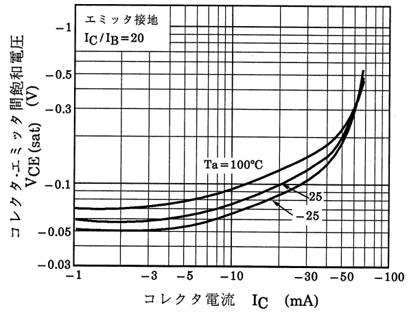
図 7.10 RN2708JE V_{CE(sat)} - I_C
