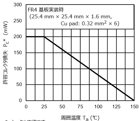
図 15.1 P_C - T_a
