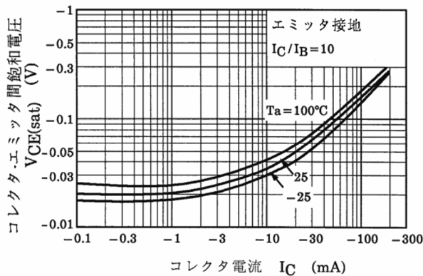
図 14.3 V_{CE(sat)} - I_C
