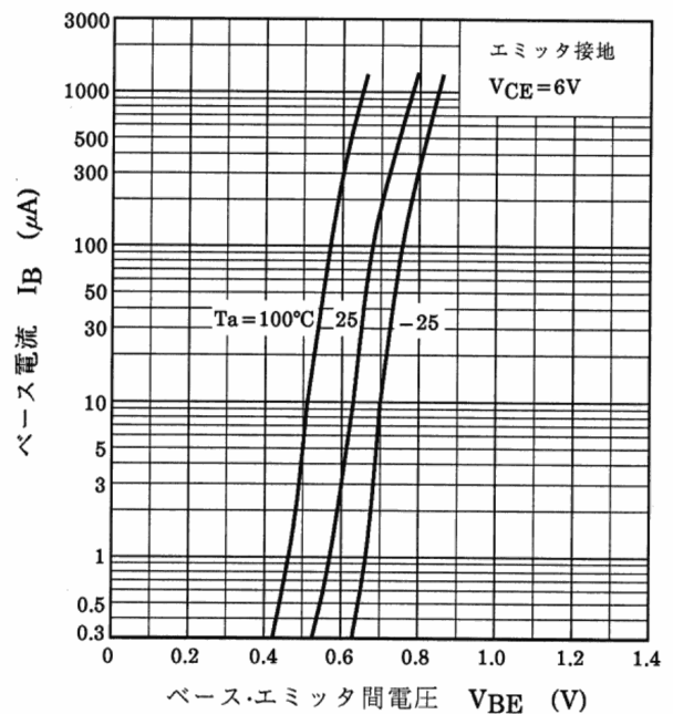
図 13.6 I_B - V_{BE}
