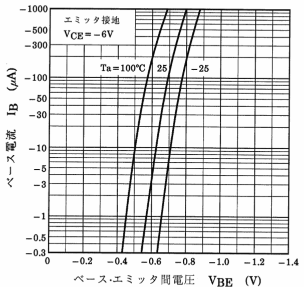
図 14.6 I_B - V_{BE}
