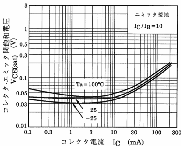
図 13.3 V_{ce(sat)} - I_c
