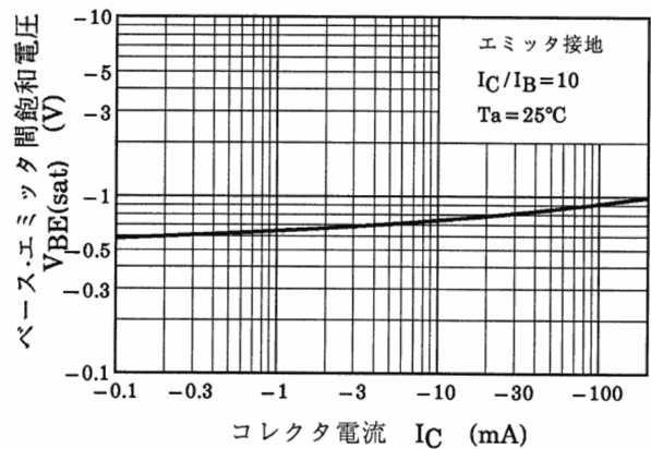
図 14.4 V_{BE(sat)} - I_C
