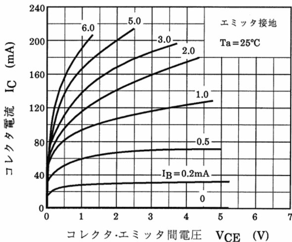
図 13.1 I_c - V_{ce}
