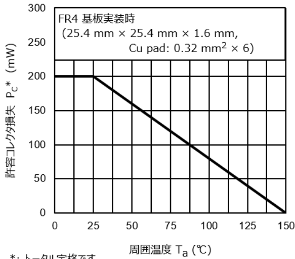
図 15.1 P_c - T_a
