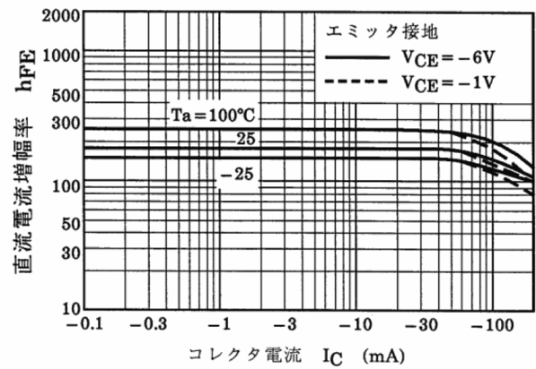
図 14.2 h_{FE} - I_C
