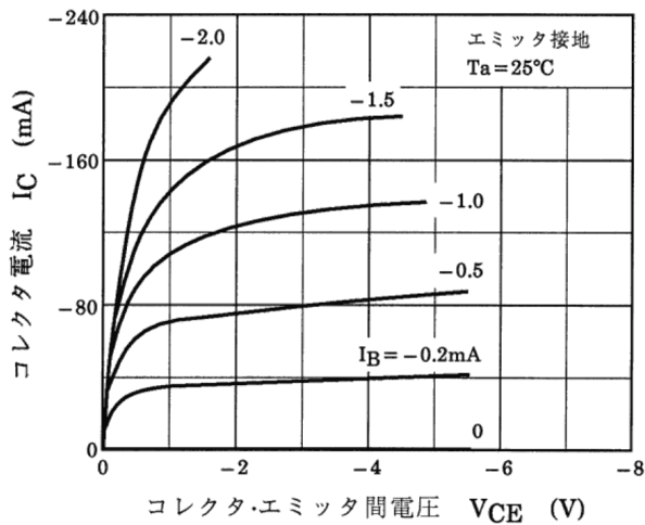
図 14.1 I_C - V_{CE}
