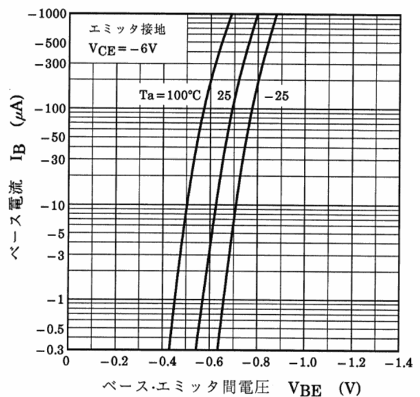
図 14.6 I_B - V_{BE}
