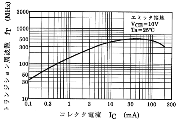
図 8.4 f_T - I_C
