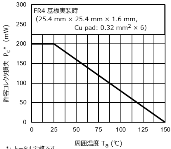
図 8.7 P_C - T_a
