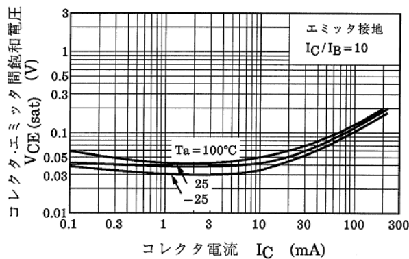
図 8.5 V_{CE(sat)} - I_C
