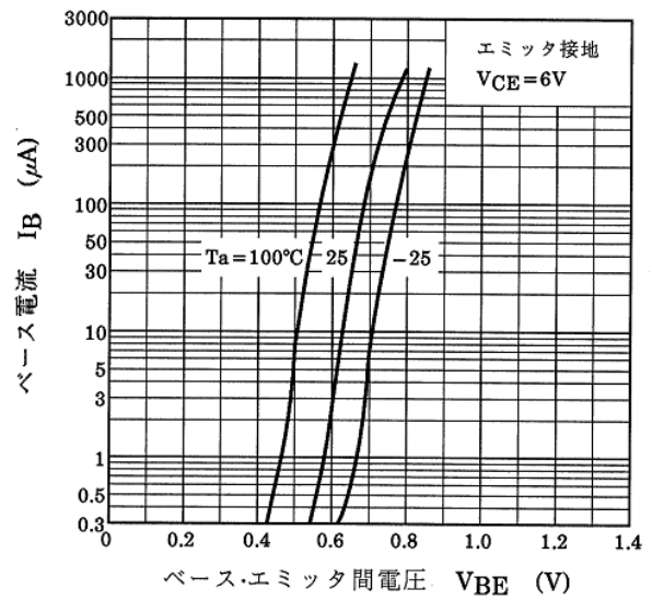
図 8.2 I_B - V_{BE}
