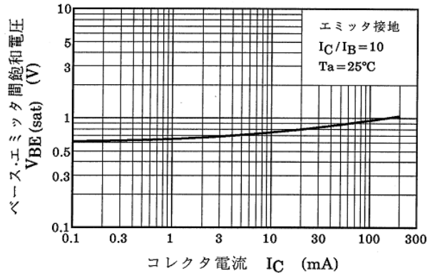
図 8.6 V_{BE(sat)} - I_C
