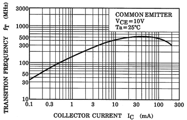
Fig. 8.4 f_T - I_C
