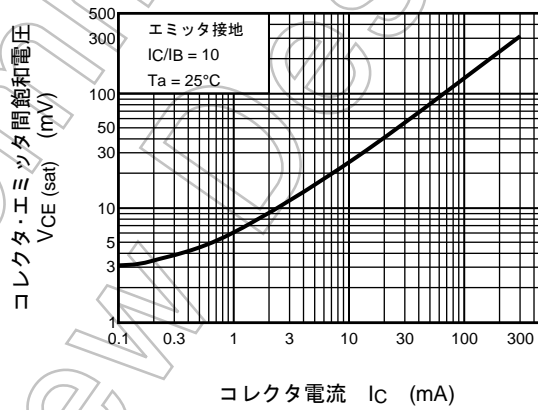
V_{CE(sat)} - I_C
