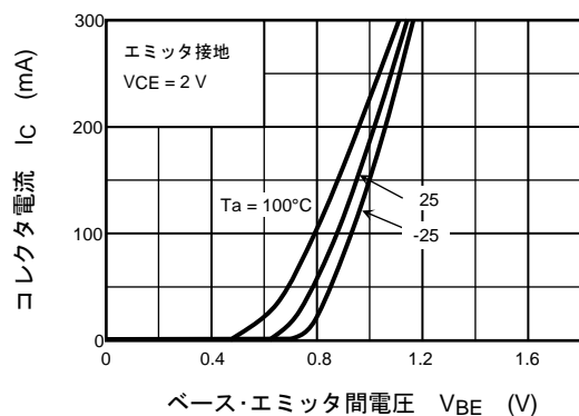
I_C - V_{BE}
