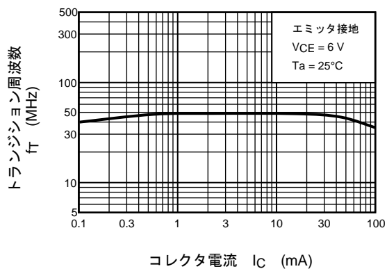
f_T - I_C
