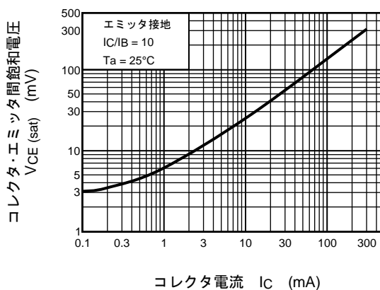
V_{CE(sat)} - I_C
