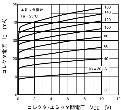
I_C - V_{CE}
