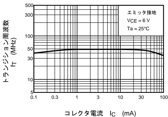
f_T - I_C
