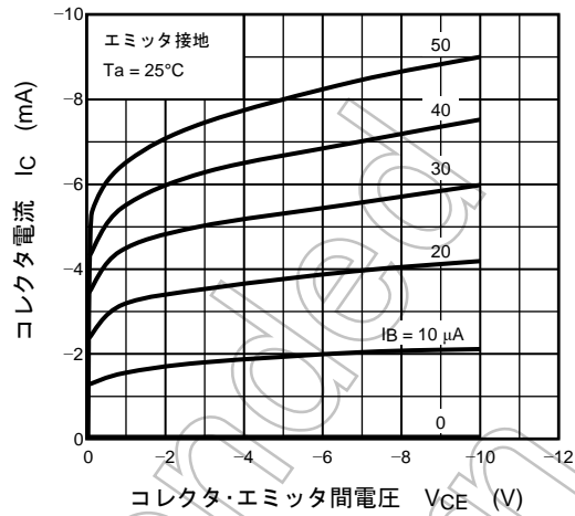
I_C - V_{CE} (逆領域)
