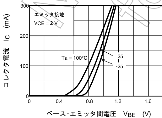
I_C - V_{BE}
