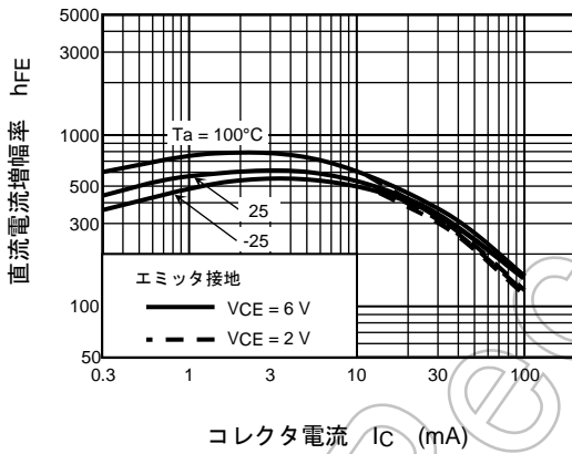
h_{FE} - I_C
