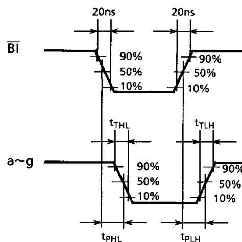
波形 4
