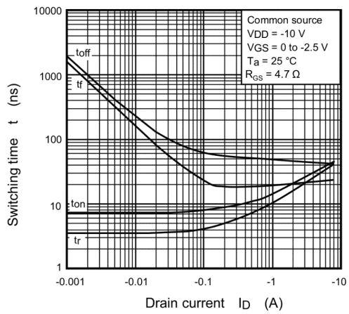
Fig. 8.10 t - I_D
