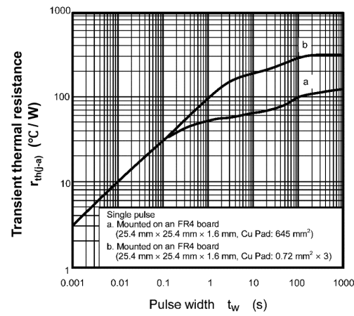
Fig. 8.12 r_{th(j-a)} - t_w
