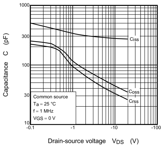
Fig. 8.9 C - V_{DS}
