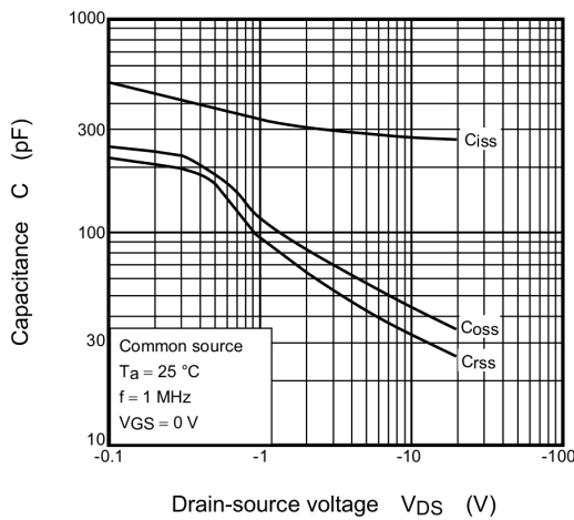
Fig. 8.9 C - V_{DS}
