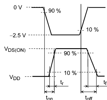
図 5.3.2 入力波形/出力波形
