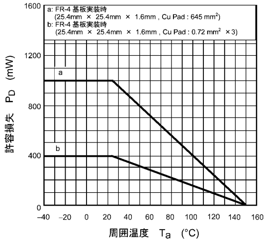
図 7.13 P_D - T_a
