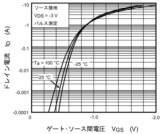
図 7.2 I_D - V_{GS}
