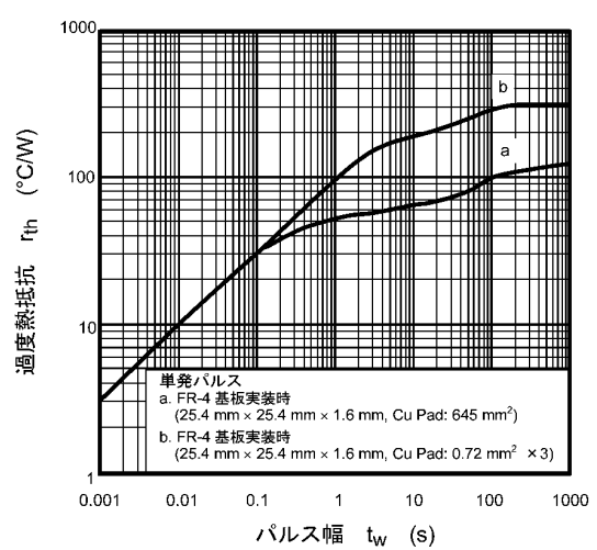
図 7.12 r_{th} - t_w
