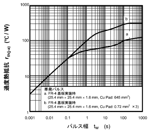
図 8.12 r_{th(j-a)} - t_w
