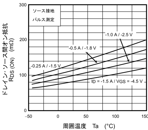
図 8.5 R_{DS(ON)} - T_a
