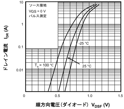
図 8.8 I_{DR} - V_{DSF}
