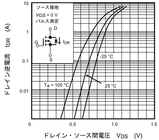
図 7.8 I_{DR} - V_{DS}
