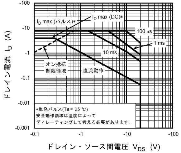
図 7.14 安全動作領域
