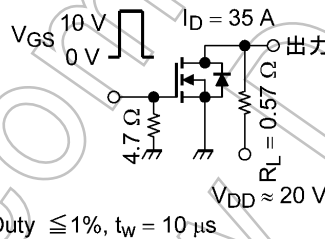
図 6.2.1 スwitchング時間の測定回路例
