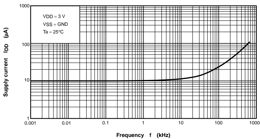
I_{DD} - f
