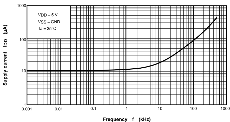
I_{DD} - f
