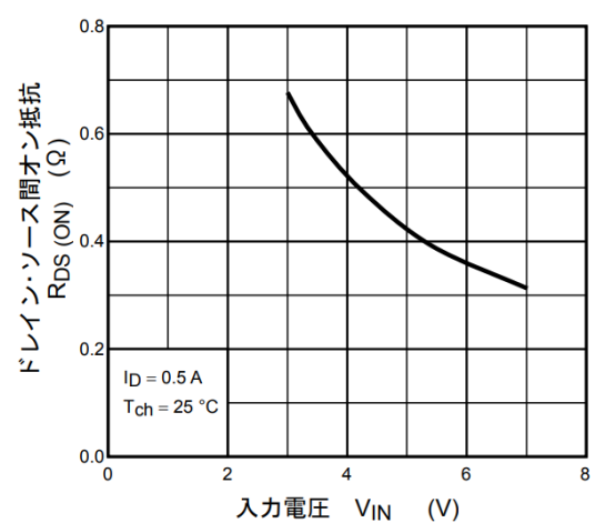
図 12.6 R_{DS(ON)} - V_{IN}
