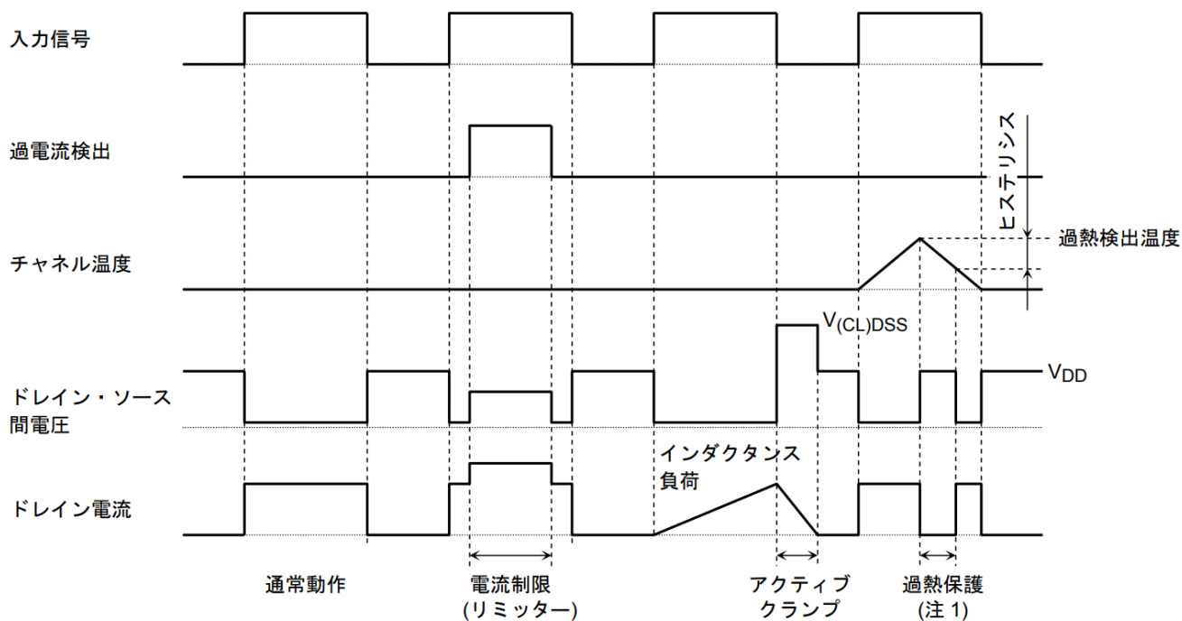
図 7.1 タイミングチャート
