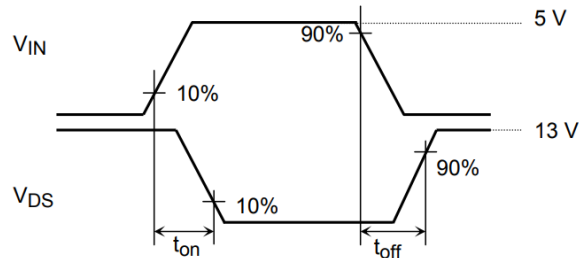
図 11.4 測定波形 2
