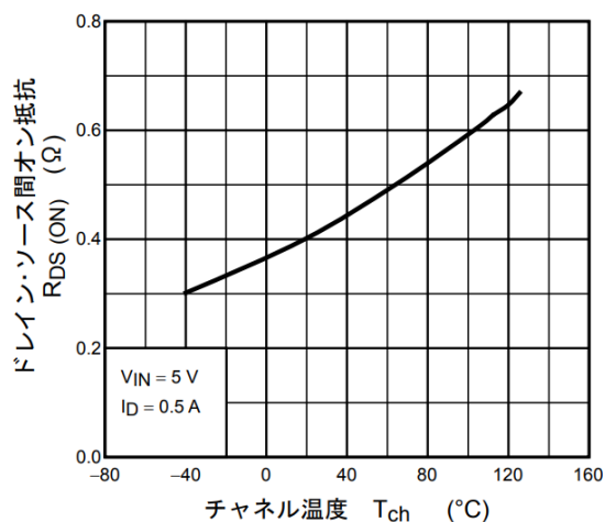
図 12.5 R_{DS(ON)} - T_{ch}
