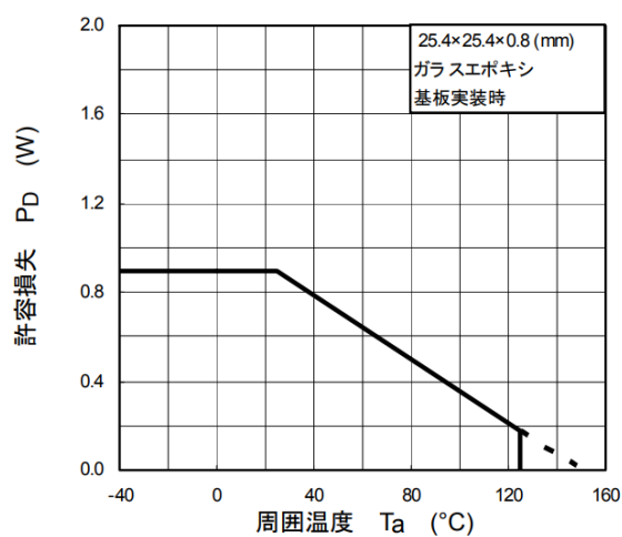
図 12.12 P_D - T_a
