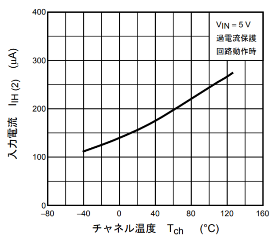
図 12.4 I_{H(2)} - T_{ch}
