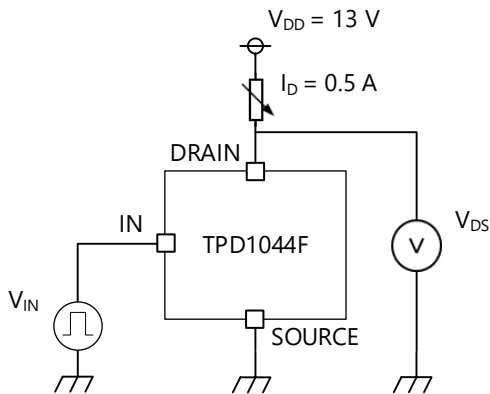
図 11.3 測定回路 2
