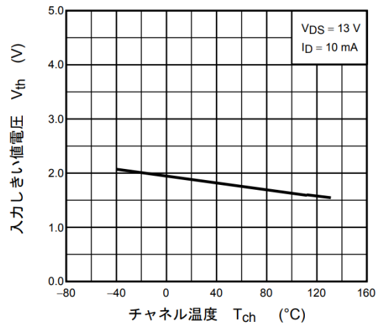
図 12.2 V_{th} - T_{ch}
