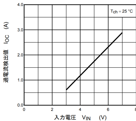
図 12.8 I_{OC} - V_{IN}
