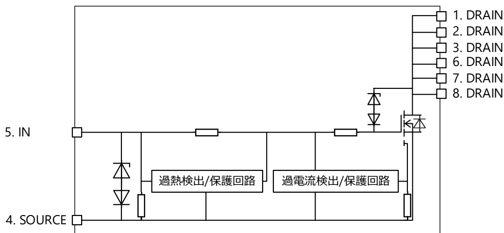
図 4.1 ブロック図
