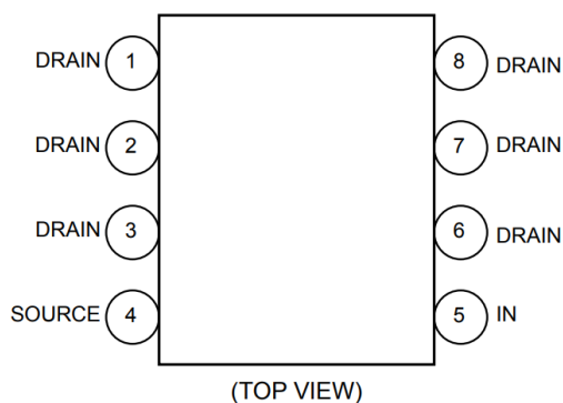
図 5.1 端子配置図 (Top view)
