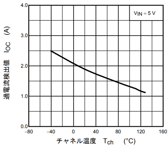
図 12.7 I_{OC} - T_{ch}
