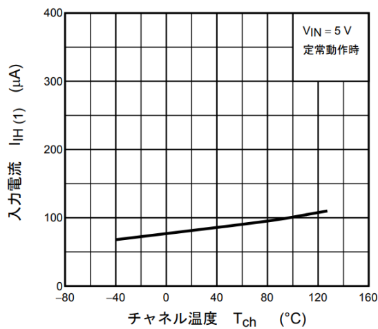
図 12.3 I_{H(1)} - T_{ch}
