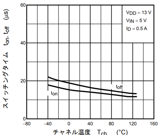
図 12.9 t_{on}, t_{off} - T_{ch}
