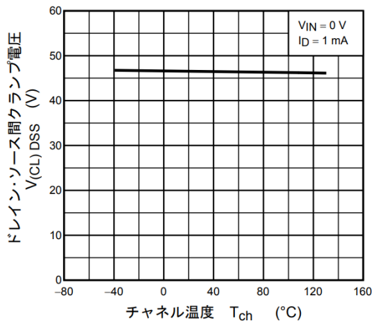
図 12.1 V_{(CL)DSS} - T_{ch}
