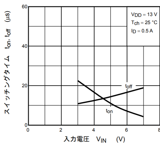
図 12.10 t_{on}, t_{off} - V_{IN}
