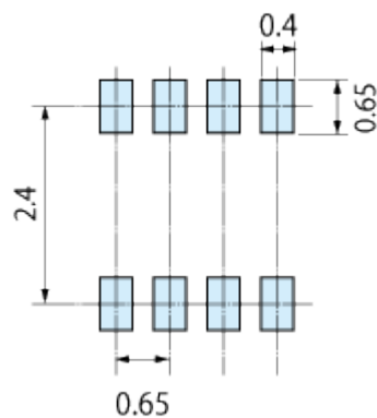
図 13.3 参考パッド寸法
