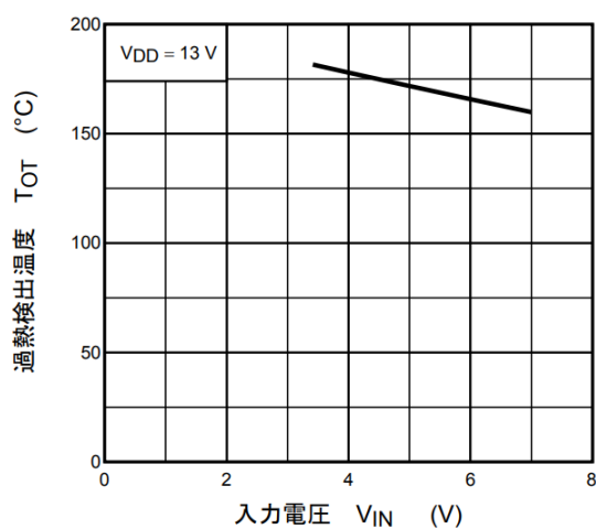
図 12.11 T_{OT} - V_{IN}
