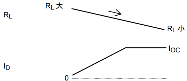
図 11.2 測定波形 1
