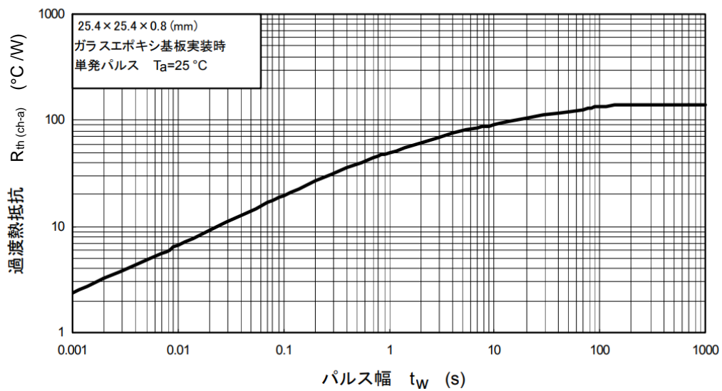
図 12.13 R_{th(ch-a)} - t_w
