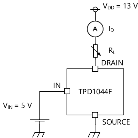
図 11.1 測定回路 1
