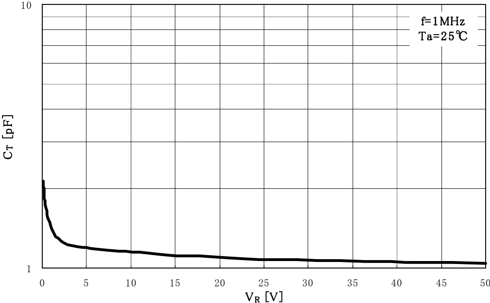
C_T-V_R
