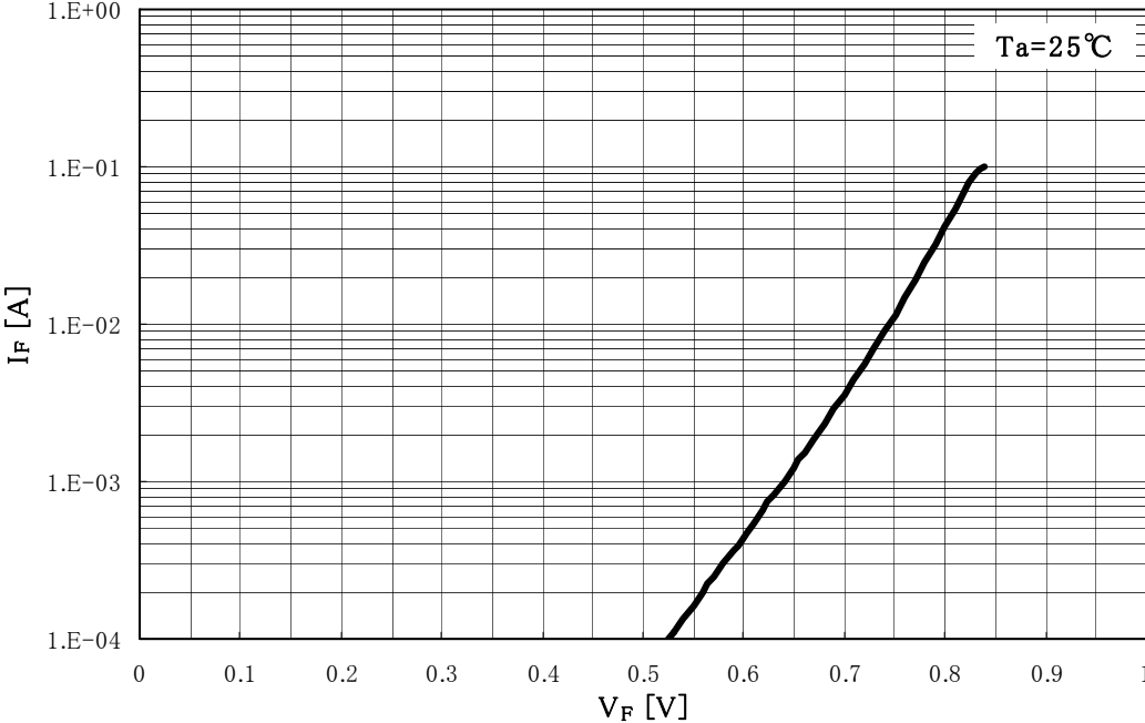
I_F-V_F
