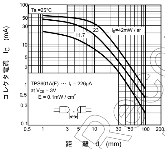
TLN108(F)との結合特性
