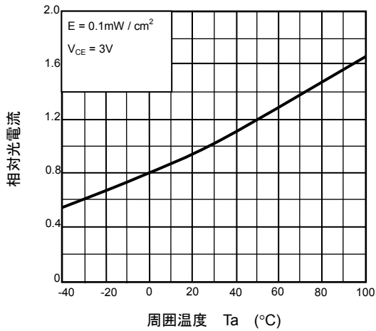
相対 I_L - T_a (標準値)
