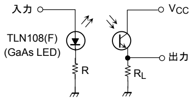
図 1. スイッチング時間測定回路
