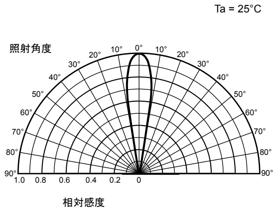
指向感度特性 (標準値)
