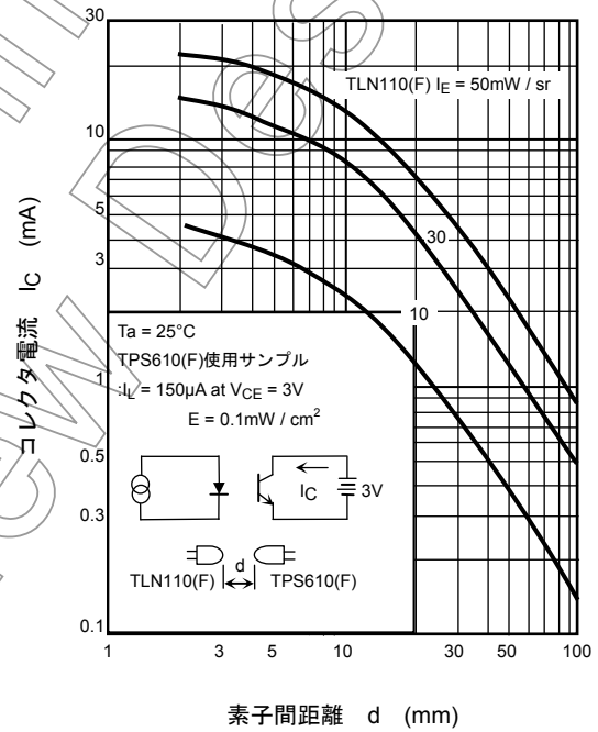
TLN110(F)との結合特性
