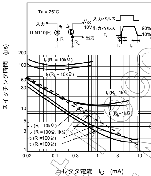
スイッチング特性 (標準値)
