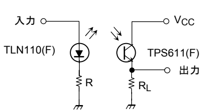
図 1. スイッチング時間測定回路
