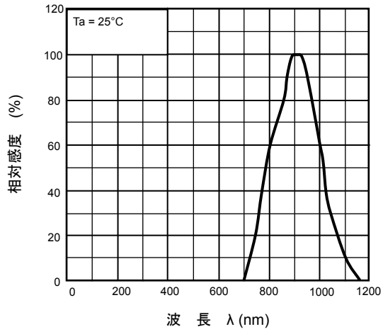
分光感度特性 (標準値)
