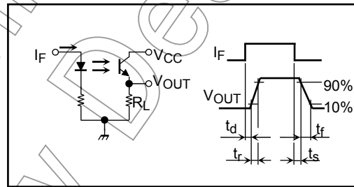
スイッチング時間の測定回路
