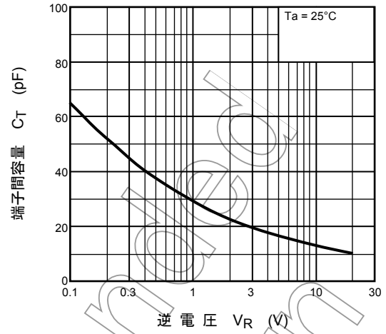
C_T - V_R (標準値)
