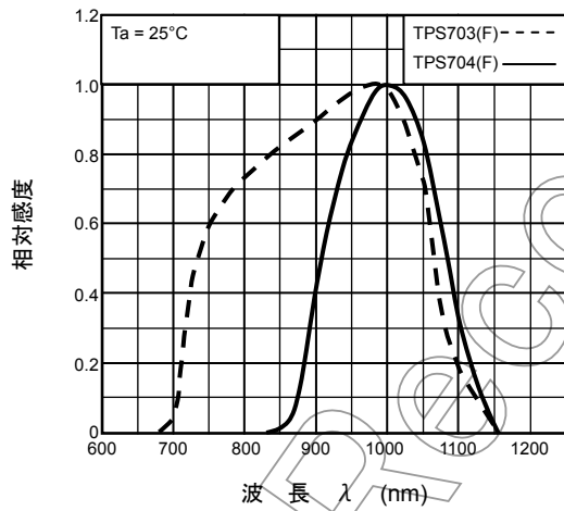
分光感度特性 (標準値)
