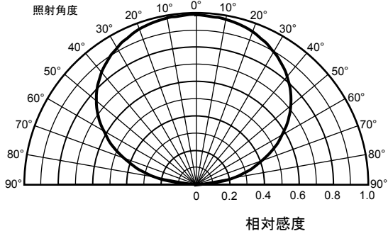
指向感度特性 (Ta = 25°C) (標準値)
