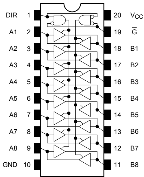
ピン接続図 (top view)
