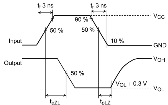
測定波形
