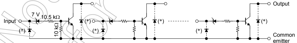
TD62502FNG
