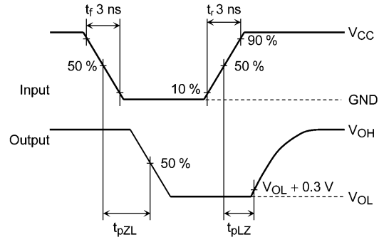
測定波形
