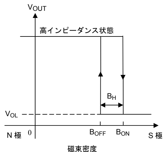
(図B) : 磁電変換特性
