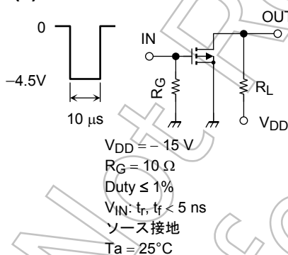
(a) 測定回路
