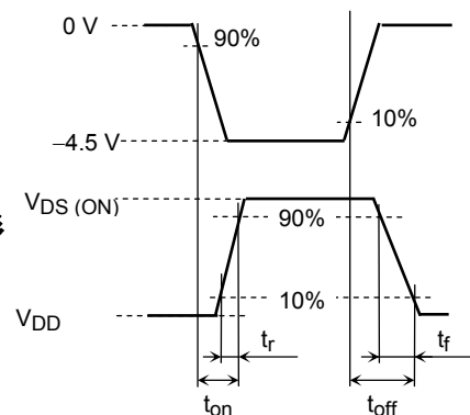
(c) 出力波形
