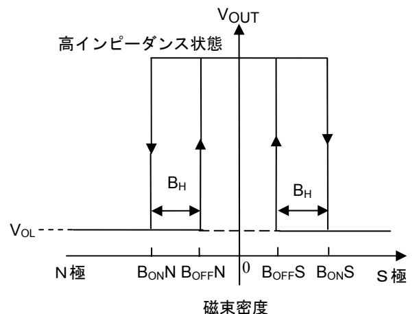
(図B): 磁電変換特性
