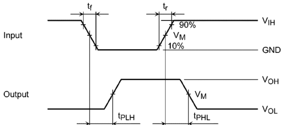
図 12.8.1 t_{PLH} , t_{PHL}
