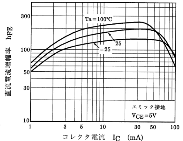
図 13.6 Q2 h_{FE} - I_C
