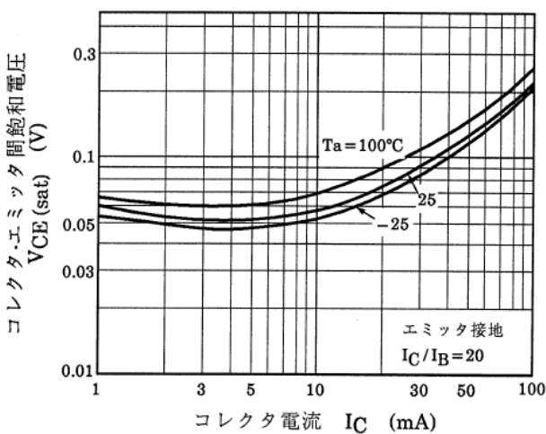
図 13.8 Q2 V_{CE(sat)}-I_C
