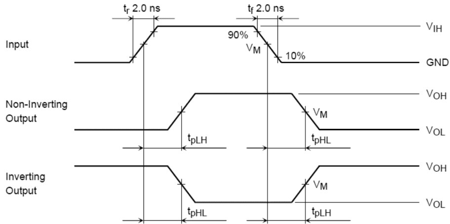
図 12.8.1 t_{pLH} , t_{pHL}
