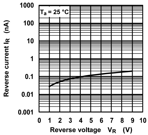
図 8.2 I_R - V_R
