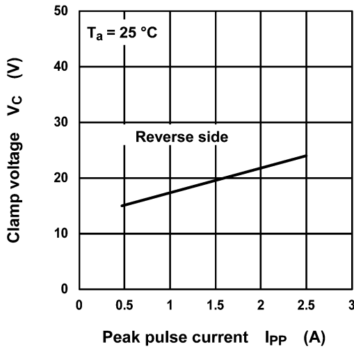
図 9.1 V_C - I_{PP}
