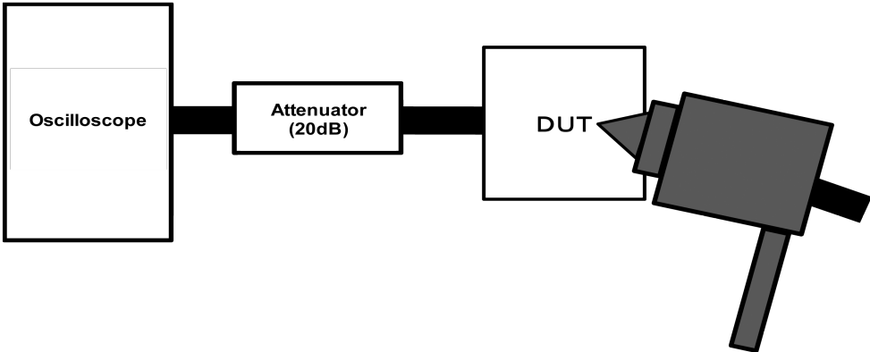
Fig. 11.3 IEC61000-4-2(Contact)
