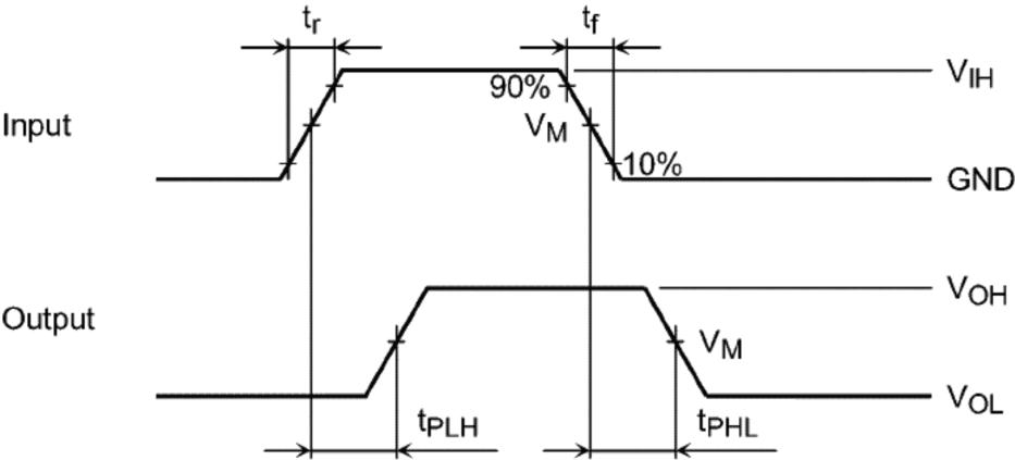
図 11.8.1 tPLH, tPHL
