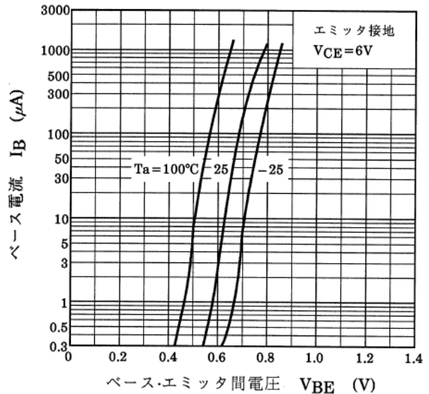
図 8.6 I_B - V_{BE}
