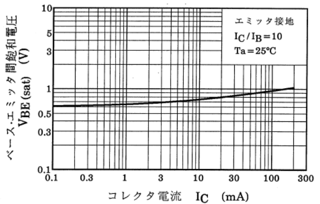
図 8.4 V_{BE(sat)} - I_C
