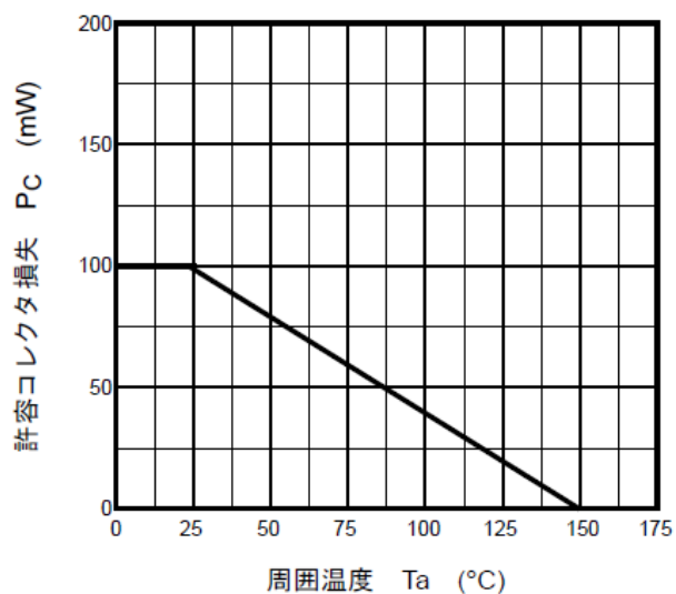
図 8.7 P_c (注1) - T_a
