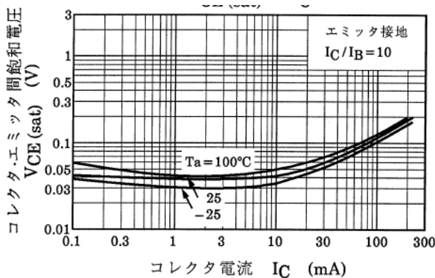
図 8.3 V_{CE(sat)} - I_C
