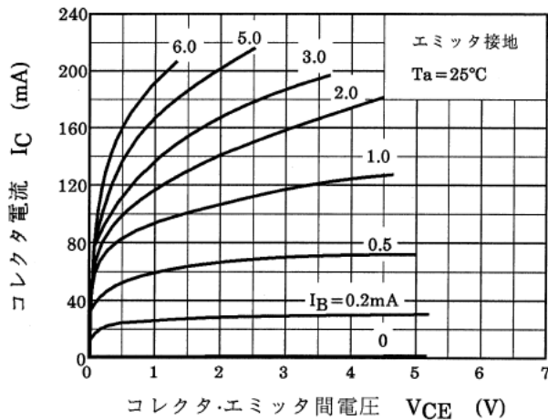
図 8.1 I_C - V_{CE}
