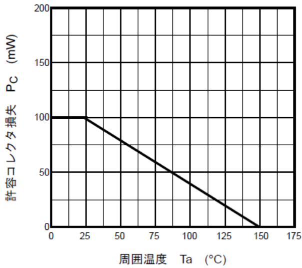
図 8.7 P_C (注1) - T_a
