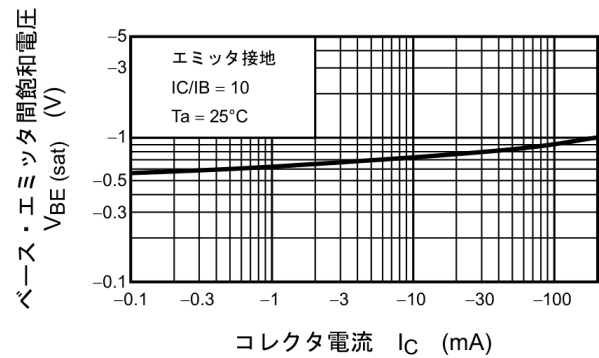
図 14.4 V_{BE(sat)} - I_C
