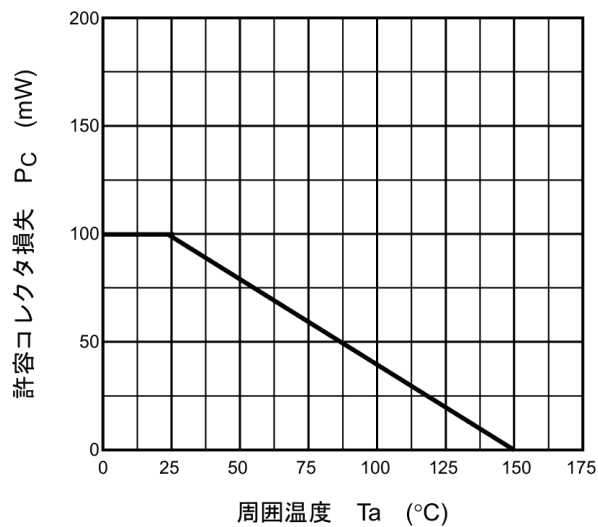
図 15.1 P_c (注1) - T_a
