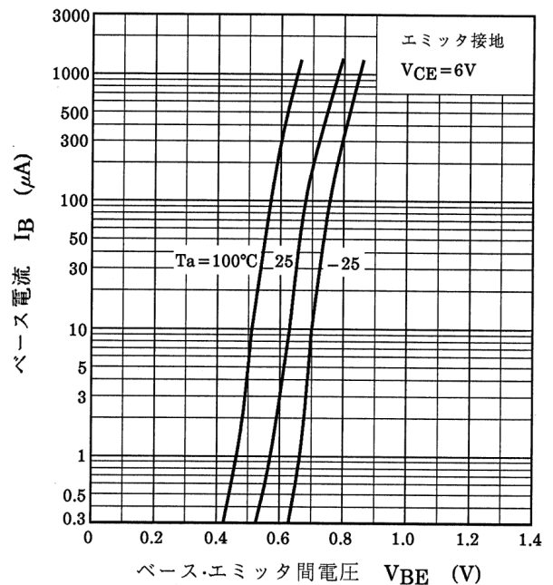
図 13.6 I_B - V_{BE}
