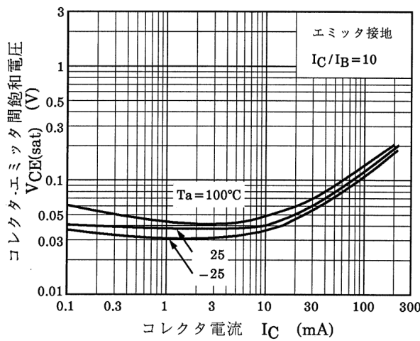
図 13.3 V_{CE(sat)} - I_C
