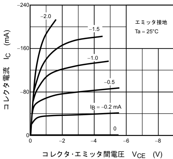
図 14.1 I_C - V_{CE}
