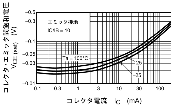
図 14.3 V_{CE(sat)} - I_C
