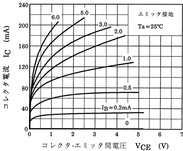
図 13.1 I_C - V_{CE}
