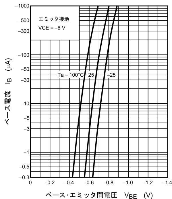
図 14.6 I_B - V_{BE}
