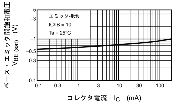
図 14.4 V_{BE(sat)} - I_C
