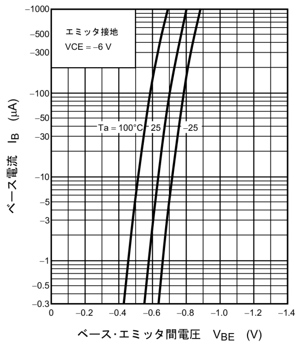
図 14.6 I_B - V_{BE}
