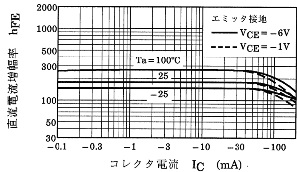
図 8.2 h_{FE} - I_C
