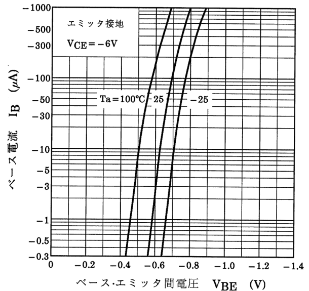
図 8.6 I_B - V_{BE}
