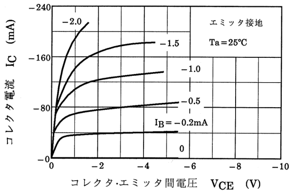
図 8.1 I_C - V_{CE}
