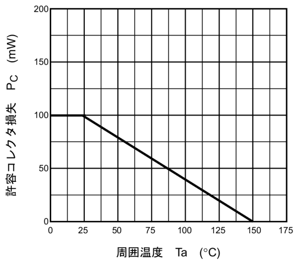
図 8.7 P_C (注1) - T_a
