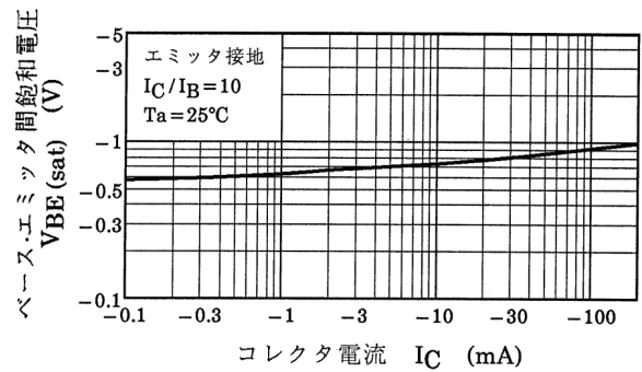
図 8.4 V_{BE(sat)} - I_C
