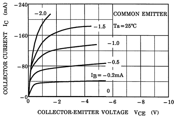
Fig. 8.1 I_C - V_{CE}
