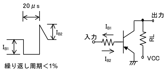
図 3. スイッチング時間測定回路
