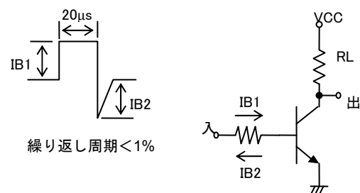
図 4. スwitchング時間測定回路
