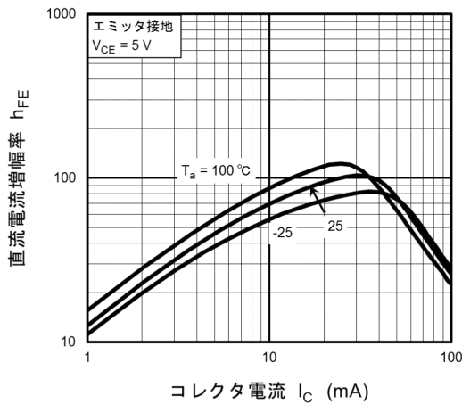
図 10.13 RN1116MFV h_{FE} - I_C
