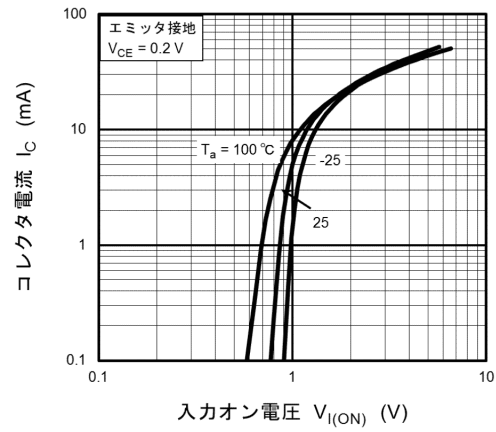
図 10.2 RN1115MFV I_C - V_{I(ON)}
