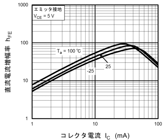
図 10.14 RN1117MFV h_{FE} - I_C
