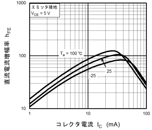
図 10.12 RN1115MFV h_{FE} - I_C
