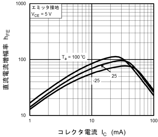
図 10.11 RN1114MFV h_{FE} - I_C
