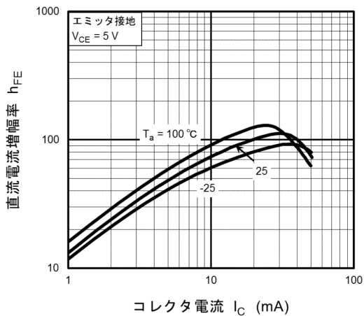
図 10.15 RN1118MFV h_{FE} - I_C
