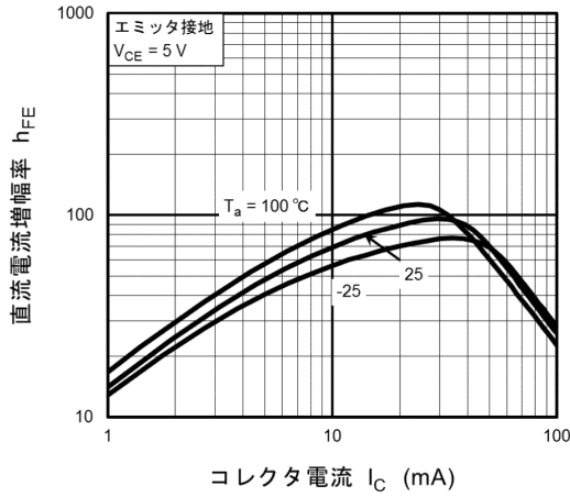
図 10.11 RN1114MFV h_{FE} - I_C
