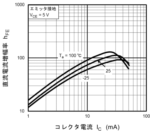
図 10.15 RN1118MFV h_{FE} - I_C
