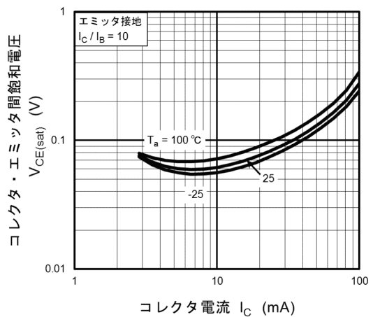
図 10.19 RN1117MFV V_{CE(sat)} - I_C
