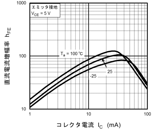
図 10.12 RN1115MFV h_{FE}-I_C
