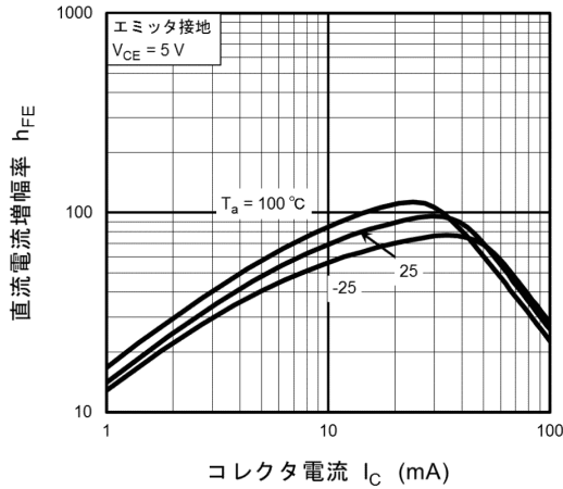
図 10.11 RN1114MFV h_{FE}-I_C
