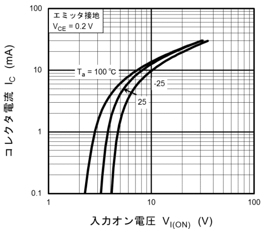
図 10.5 RN1118MFV I_C - V_{I(ON)}
