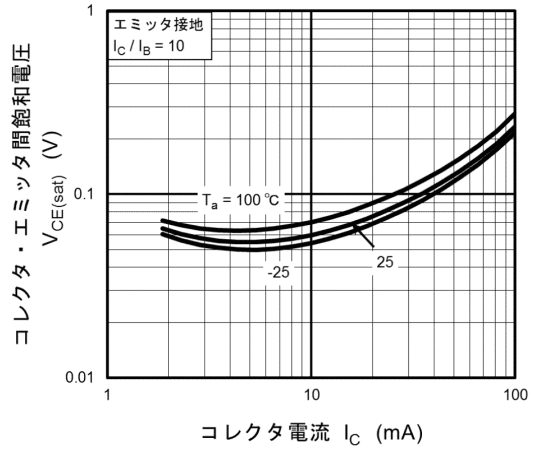
図 10.17 RN1115MFV V_{CE(sat)} - I_C
