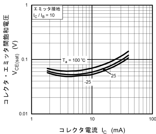
図 10.20 RN1118MFV V_{CE(sat)} - I_C
