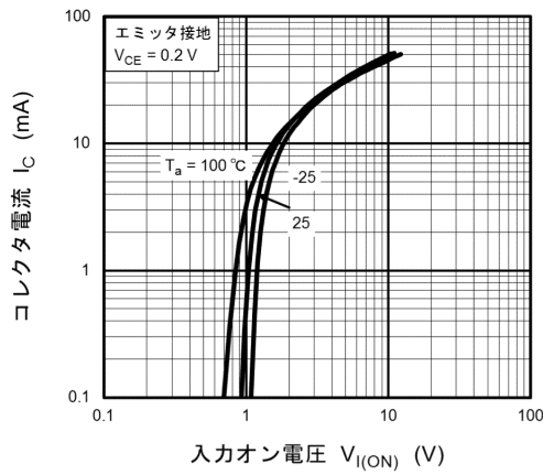
図 10.3 RN1116MFV I_C - V_{I(ON)}
