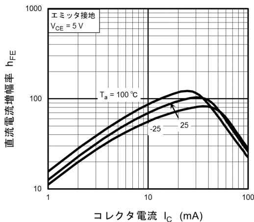
図 10.13 RN1116MFV h_{FE}-I_C
