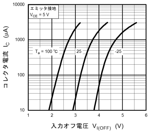
図 10.10 RN1118MFV I_C - V_{I(OFF)}
