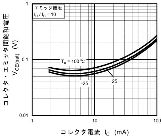
図 10.16 RN1114MFV V_{CE(sat)} - I_C
