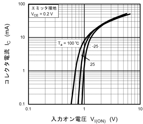
図 10.2 RN1115MFV I_C - V_{I(ON)}
