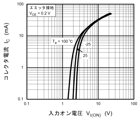
図 10.4 RN1117MFV I_C - V_{I(ON)}
