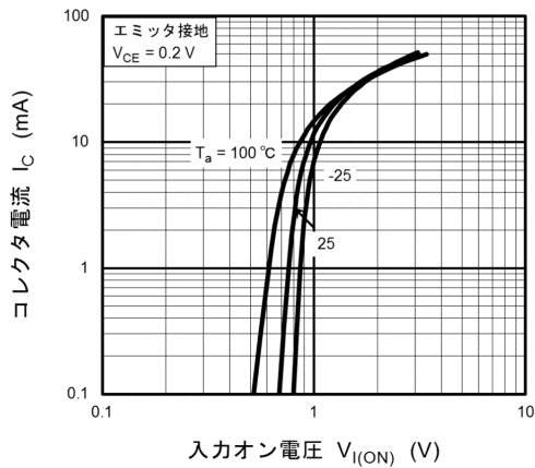
図 10.1 RN1114MFV I_C - V_{I(ON)}
