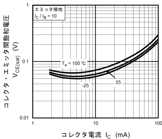
図 10.18 RN1116MFV V_{CE(sat)} - I_C
