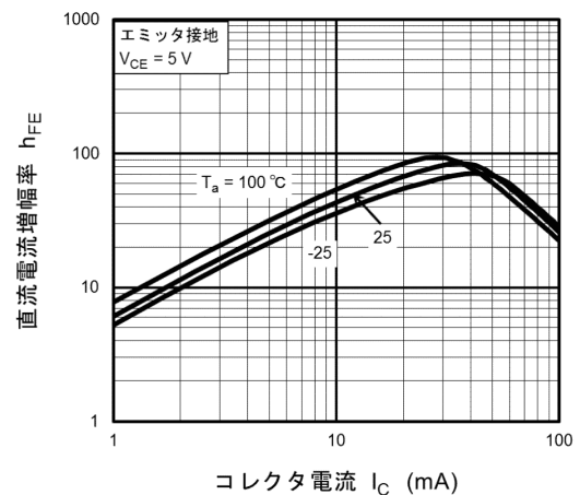
図 10.14 RN1117MFV h_{FE}-I_C
