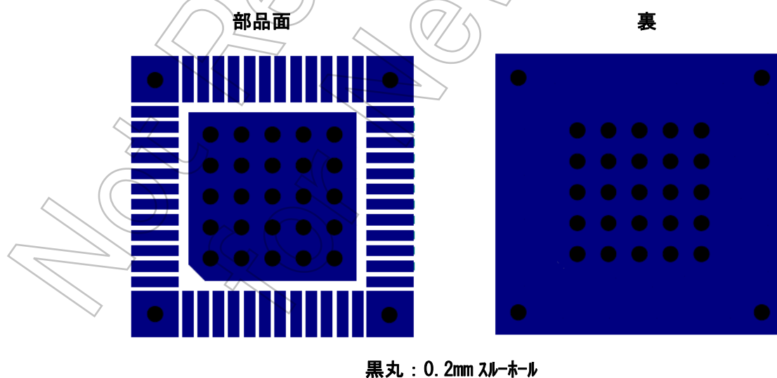
フットパターン例(両面基板)
