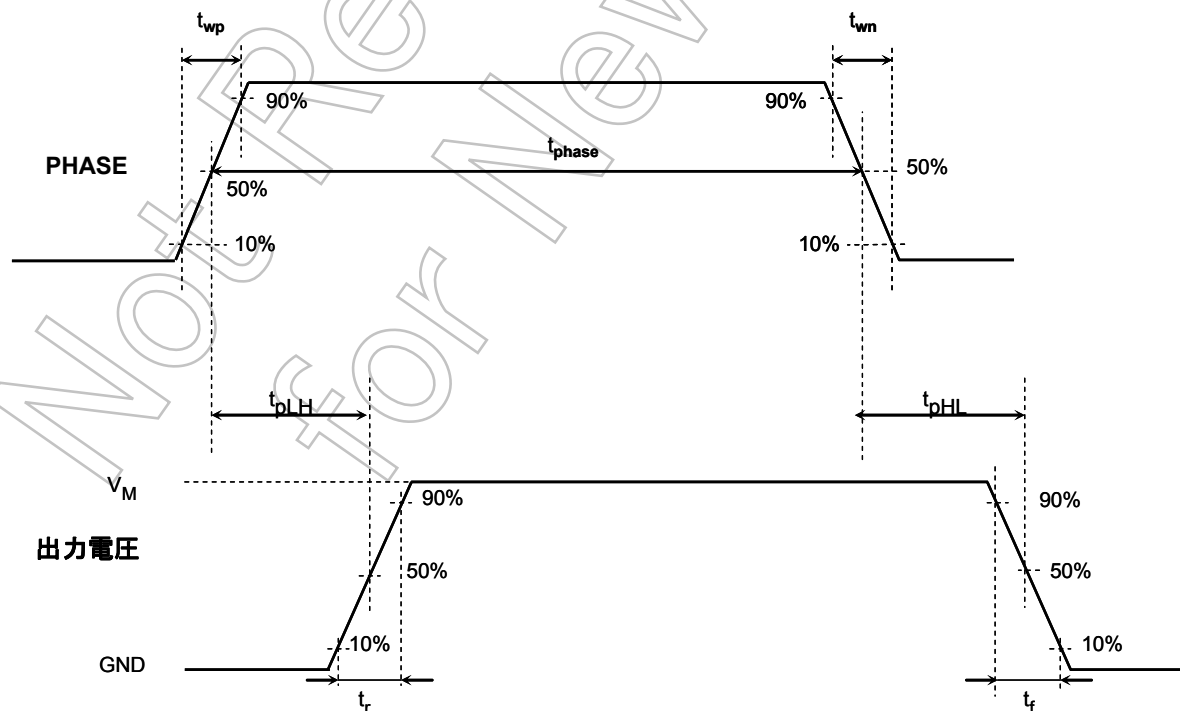
出力トランジスタ・スイッチング特性のタイミング
