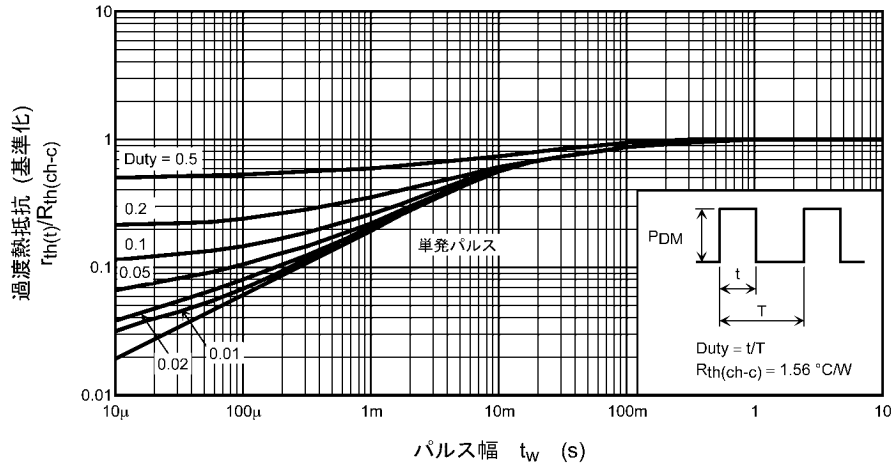
図 8.13 r_{th}(t)/R_{th}(ch-c) - t_w (最大値 (保証値))
