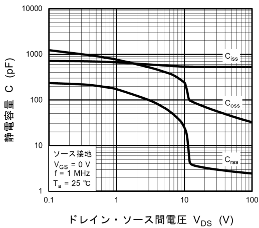
図 8.9 C - V_{DS}
