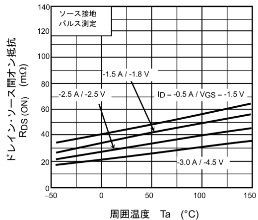
図 7.6 R_{DS(ON)} - T_a
