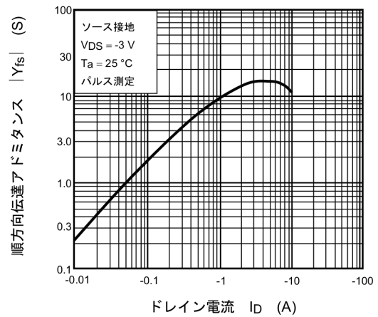
図 7.8 |Y_{fs}| - I_D
