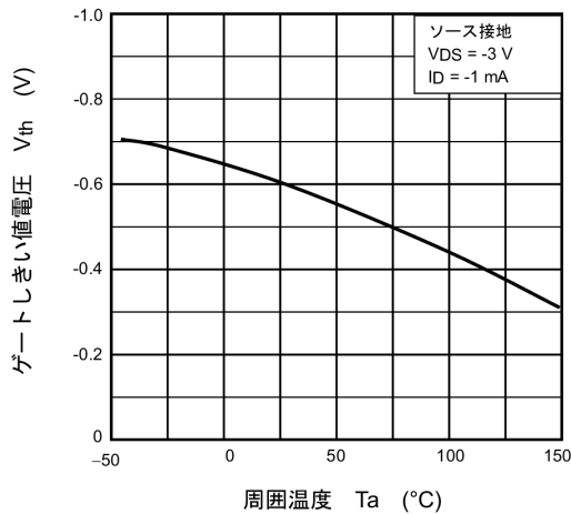
図 7.7 V_{th} - T_a
