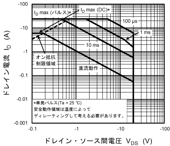
図 7.15 安全動作領域
