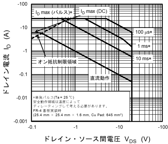
図 8.15 安全動作領域
