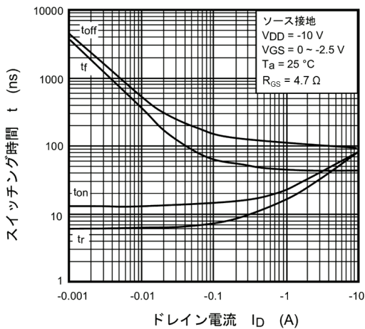
図 8.11 t - I_D
