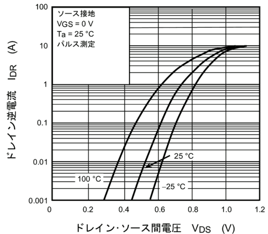
図 8.12 I_{DR} - V_{DS}
