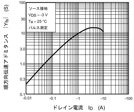
図 8.8 |Y_{fs}| - I_D
