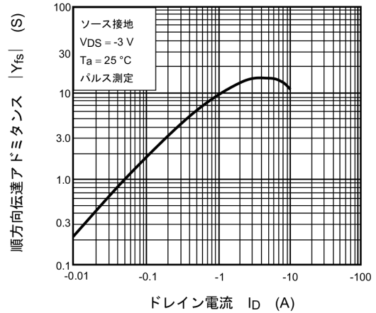
図 8.8 |Y_{fs}| - I_D
