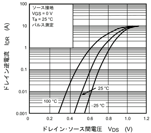
図 8.12 I_{DR} - V_{DS}
