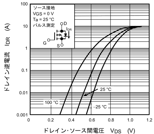
図 7.12 I_{DR} - V_{DS}
