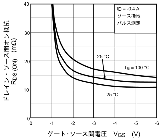
図 7.3 R_{DS(ON)} - V_{GS}
