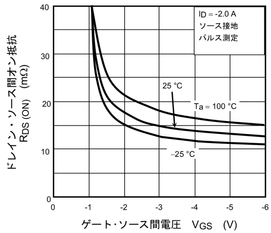
図 7.4 R_{DS(ON)} - V_{GS}
