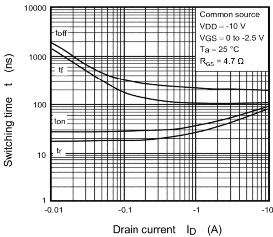
Fig. 7.11 t - I_D
