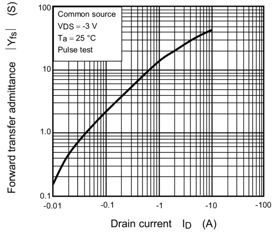
Fig. 7.8 |Y_{fs}| - I_D
