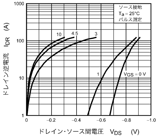
図 8.7 I_{DR} - V_{DS}
