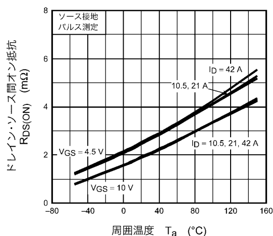
図 8.6 R_{DS(ON)} - T_a
