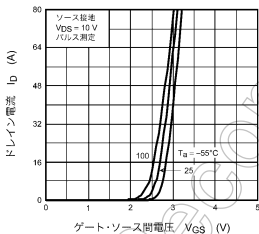
図 8.3 I_D - V_{GS}
