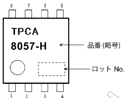
図 7.1 現品表示
