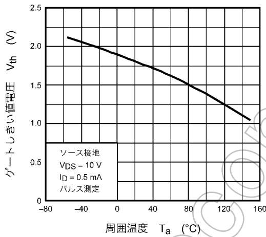
図 8.9 V_{th} - T_a
