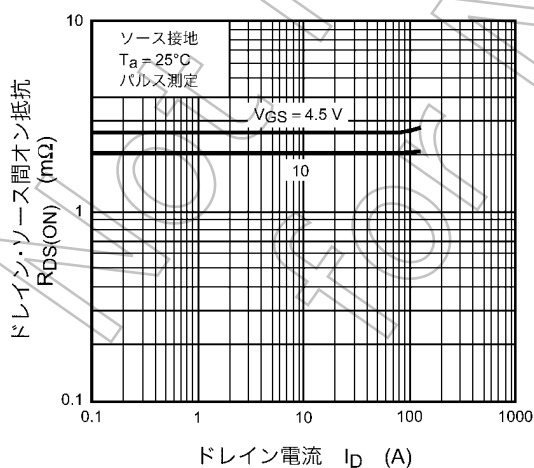
図 8.5 R_{DS(ON)} - I_D
