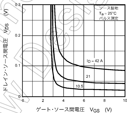
図 8.4 V_{DS} - V_{GS}
