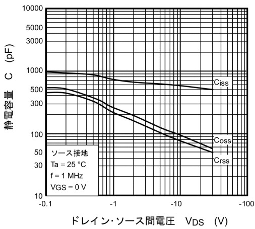
図 8.9 C - V_{DS}
