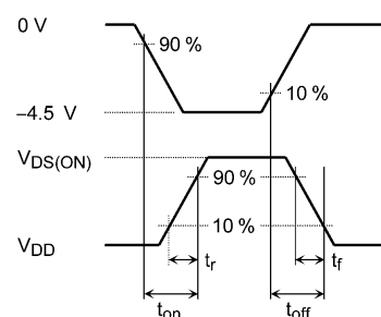
図 6.3.2 入力波形/出力波形
