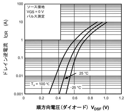
図 8.12 I_{DR} - V_{DSF}
