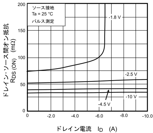
図 8.5 R_{DS(ON)} - I_D
