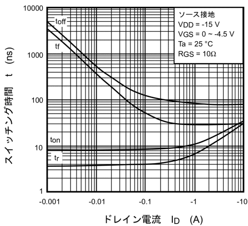
図 8.11 t - I_D
