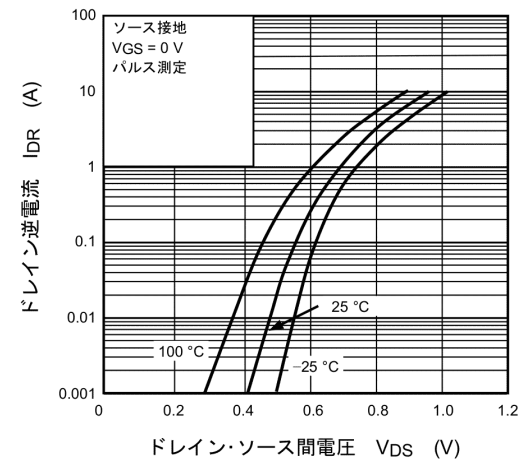
図 8.12 I_{DR} - V_{DS}
