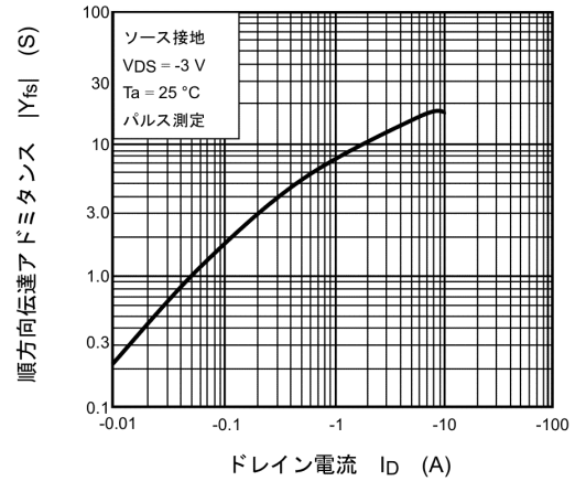
図 8.8 |Y_{fs}| - I_D
