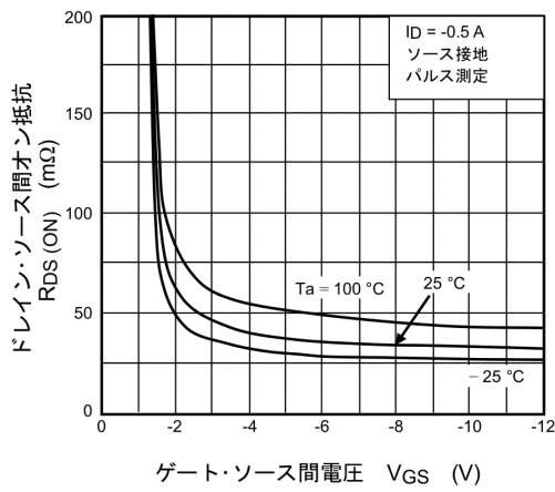
図 8.3 R_{DS(ON)} - V_{GS}
