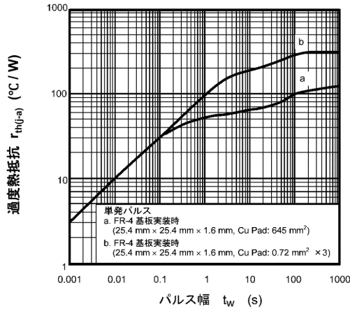
図 8.13 r_{th(j-a)} - t_w
