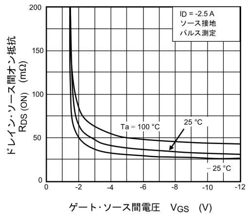
図 8.4 R_{DS(ON)} - V_{GS}
