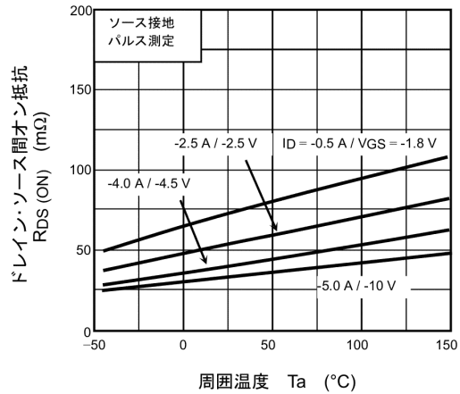
図 8.6 R_{DS(ON)} - T_a
