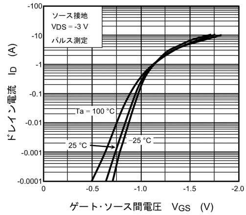
図 8.2 I_D - V_{GS}
