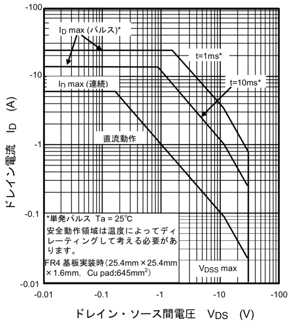
図 8.15 安全動作領域
