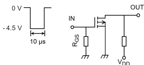
図 6.3.1 スwitchング時間の測定回路
