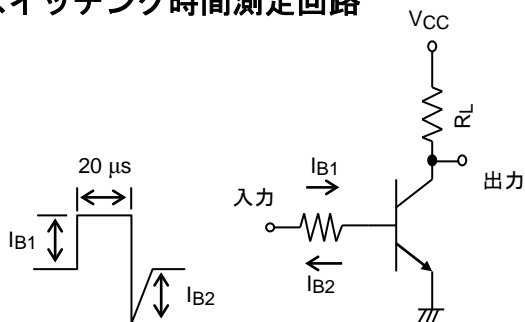
図 3. スwitching時間測定回路
