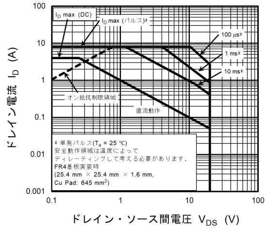
図 9.14 安全動作領域
