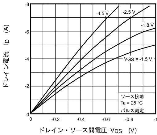
図 9.1 I_D - V_{DS}
