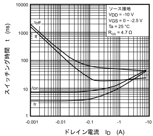
図 9.10 t - I_D
