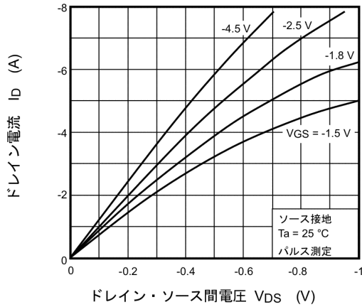
図 9.1 I_D - V_{DS}
