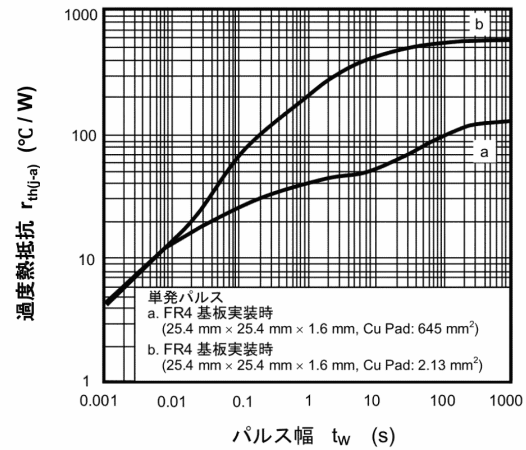
図 9.12 r_{th(j-a)} - t_w
