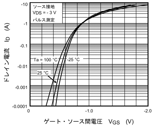
図 9.2 I_D - V_{GS}
