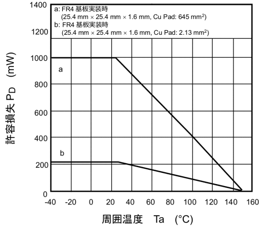
図 9.13 P_D - T_a
