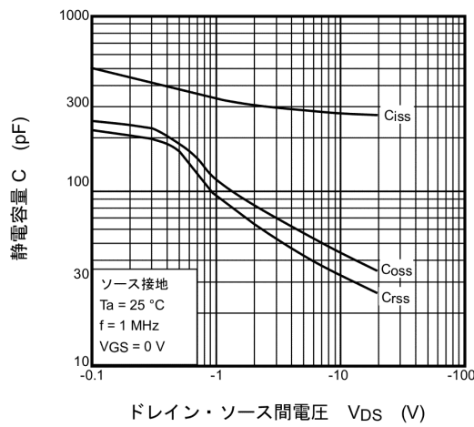
図 9.9 C - V_{DS}
