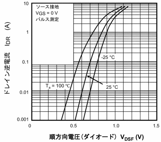
図 9.8 I_{DR} - V_{DSF}
