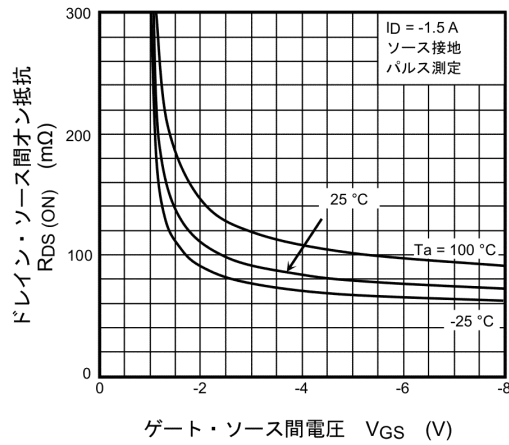
図 9.3 R_{DS(ON)} - V_{GS}
