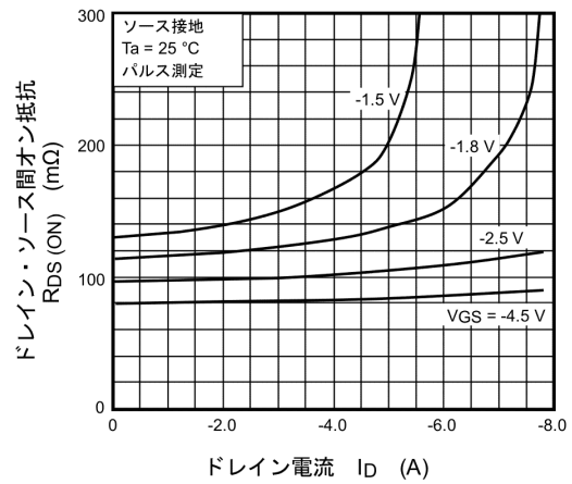
図 9.4 R_{DS(ON)} - I_D
