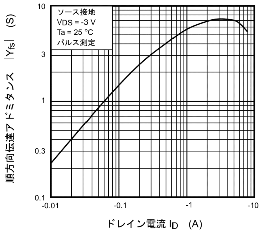
図 9.7 |Y_{fs}| - I_D
