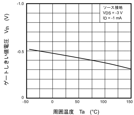
図 9.6 V_{th} - T_a
