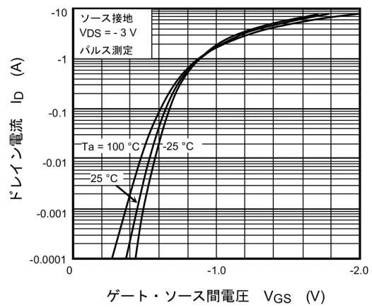
図 9.2 I_D - V_{GS}
