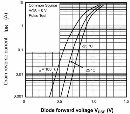
Fig. 9.8 I_{DR} - V_{DSF}
