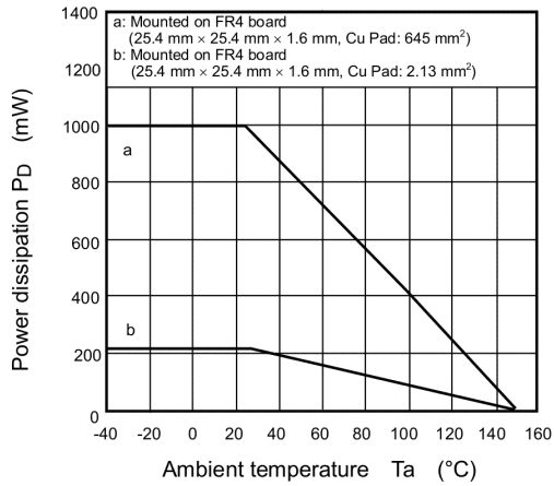
Fig. 9.13 P_D - T_a
