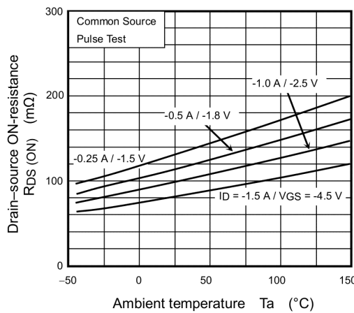
Fig. 9.5 R_{DS(ON)} - T_a
