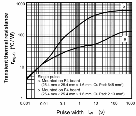
Fig. 9.12 r_{th(j-a)} - t_w
