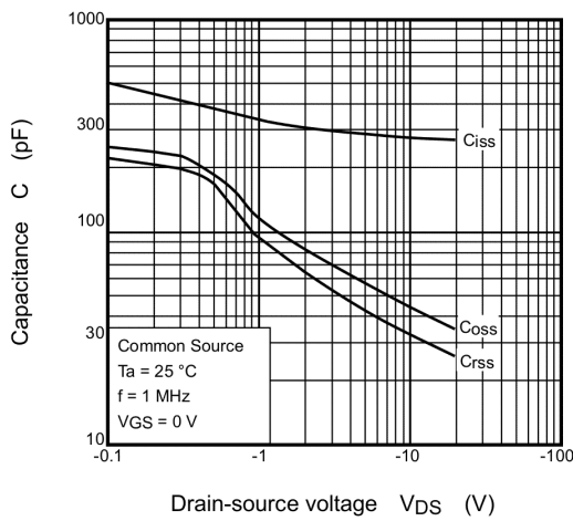
Fig. 9.9 C - V_{DS}
